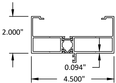
7 DOOR JAMB
