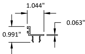
35 DOOR STOP
