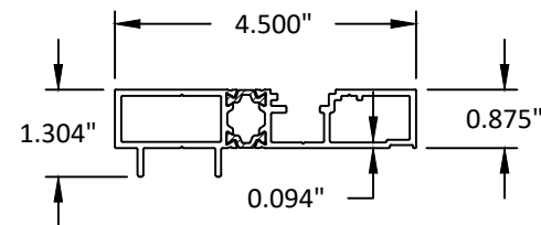
34 THERMAL JAMB SUBFRAME (POCKET)
