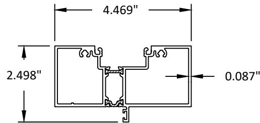
8 TRANSOM BAR
